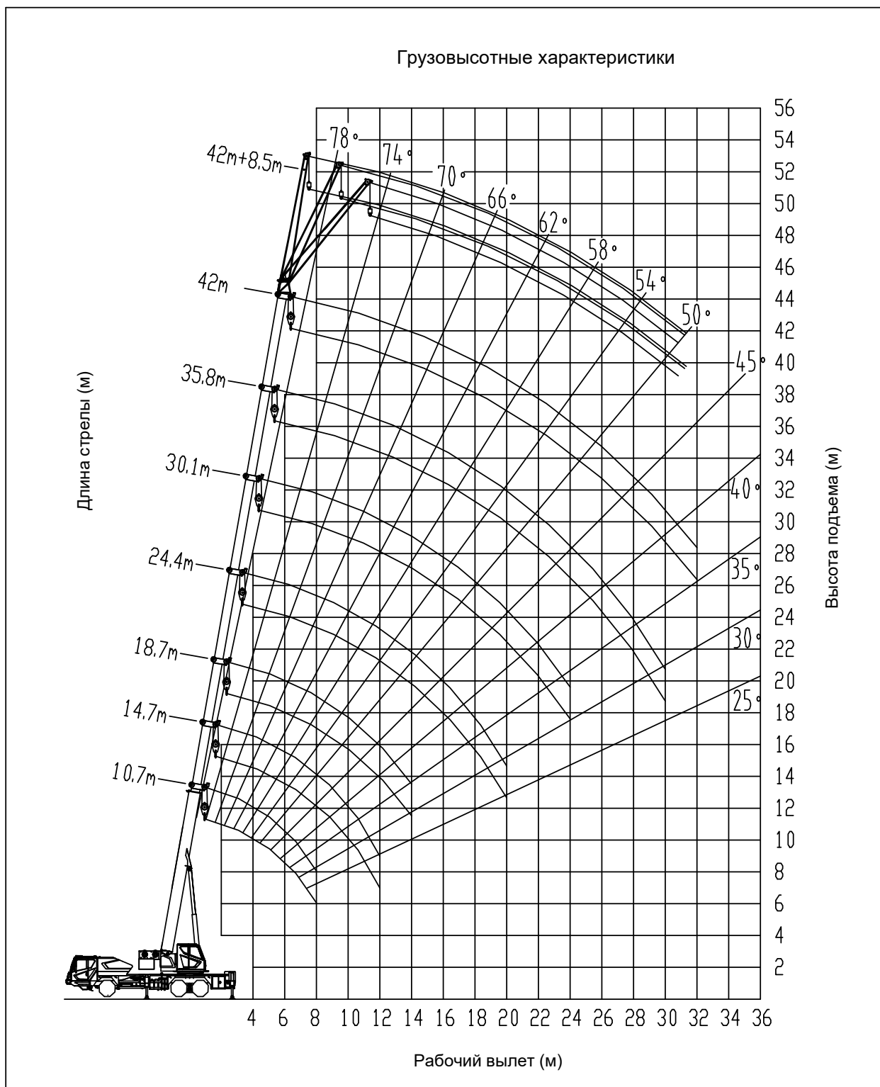
Рисунок 1 Грузовысотные характеристики
